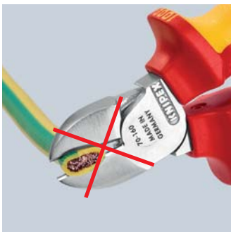
Рез кабеля диагональными кусачками: большое усилие, неаккуратный рез, сильная деформация и смятие кабеля
