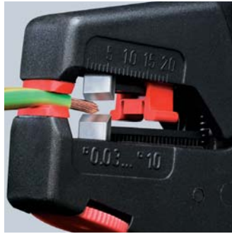
12 40 200: прецизионное удаление изоляции без повреждения проводника
