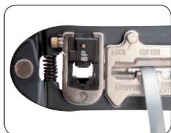
Обрезка провода
