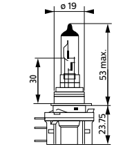
H15
