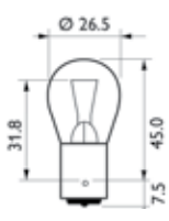
P21W
