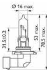
HB3
