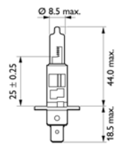
H1
