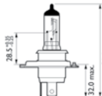
H4
