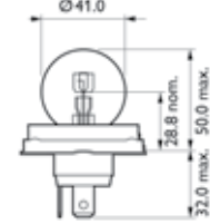
R2
