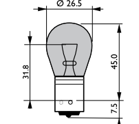
PY21W
