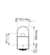
R5W
