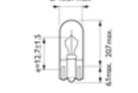
W2,2W-W2,5W W3W-W5W(Y)
