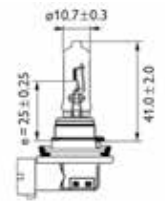
H9
