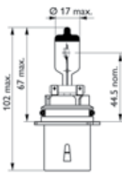
HB5
